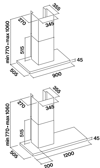
Versión 120 cm disponible solo con tubo desplazado a la izquierda
