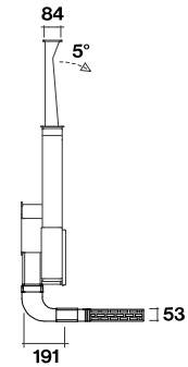
Vista lateral motor Slim en la parte trasera y filtro en zocalo Slim KACL.951 h60
