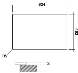
Medidas de encastre (M1/M2)
