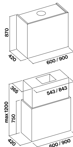
versión panelable. la botonera esta situada en la parte inferior de la campana.
