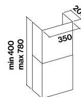
Alargo opcional
