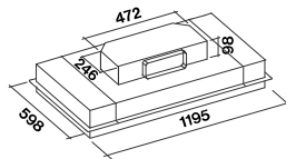
Motor SLIM (exclusivamente sobre chasis)
