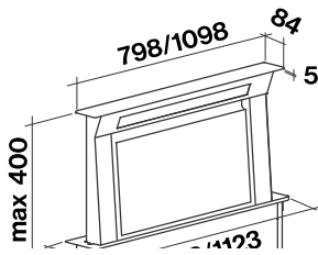
Medidas de encastre 90 cm: 98 mm x 810 mm 120 cm: 98 mm x 1110 mm
