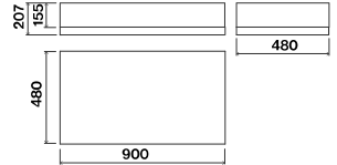
Versión Mural
