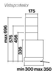
Alargo opcional
