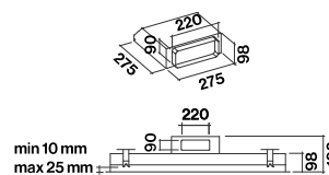
Vista lateral con unión
