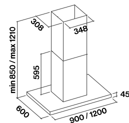
Mural. Sin tubo decorativo superior H560 mm / con tubo superior H min 770mm - max 1060 mm Isla. Sin tubo decorativo superior H 640 mm / con tubo superior H min 850 mm - max 1210 mm
