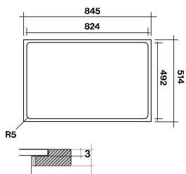
Medidas para enrase (M1/M2)
